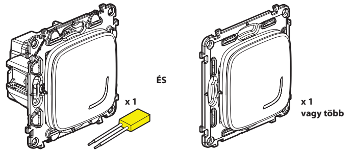
Intelligens fényerő szabályozó kapcsoló + kompenzátor (a csomag nem tartalmazza)
